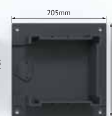
Platine au sol Floor Plate
