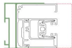
Führungsschienen 56 / coulisses 56
