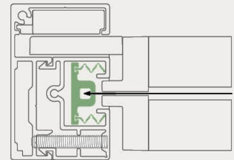
Detailansicht Zip / détail Zip
